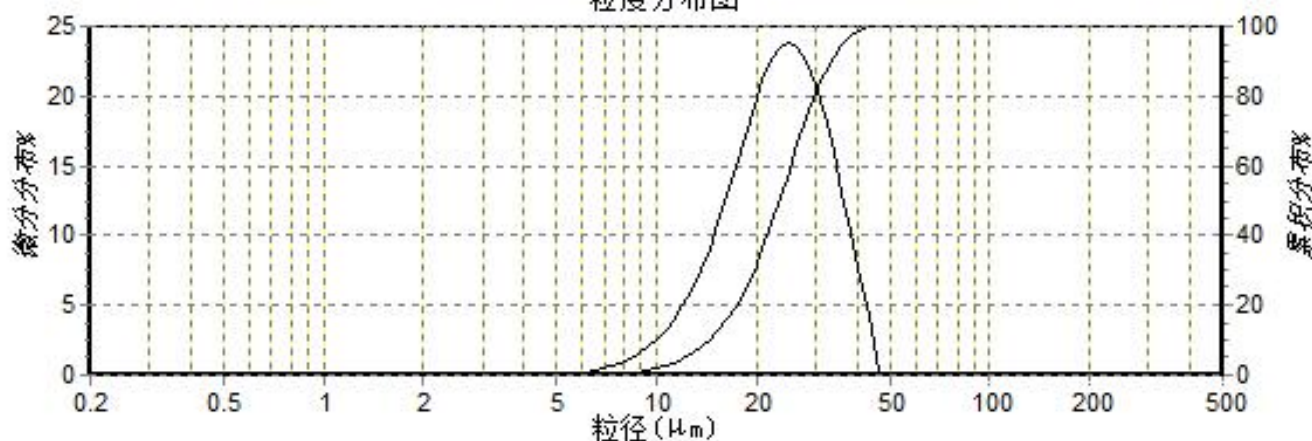
粒度分布图
